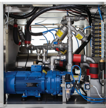
Быстрое и экономное прохождение циклов благодаря двухступенчатому вакуумному насосу
