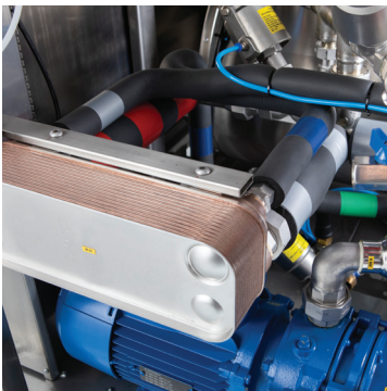
Изолированные трубы имеют цветовую кодировку.
